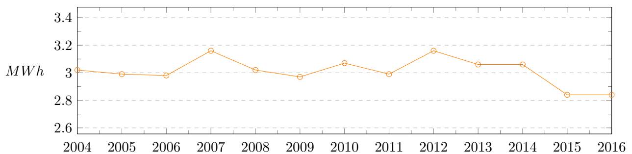
Figura 5: Variación interanual de la generación fotovoltaica.
